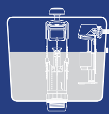
VÁLVULA DE ENTRADA EN POSICIÓN CERRADA
