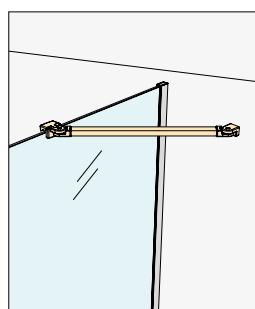
Angular à parede
