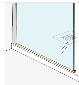
Perfil ao chão de vidro fixo de 8mm
