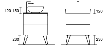
PÉS PARA LAVATÓRIOS DE POUSAR/ VENETO ALTURA 230 mm
