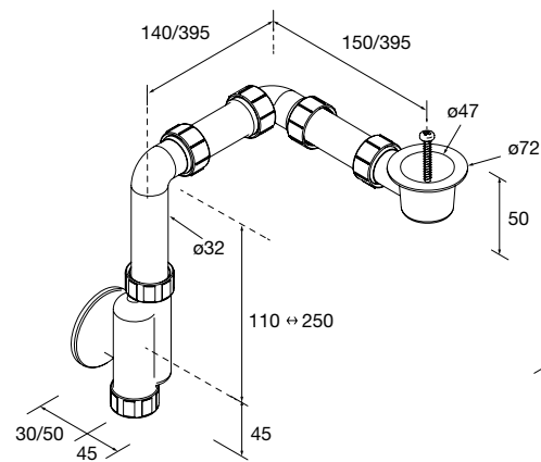
SIFÃO REDUZIDO CONEX
