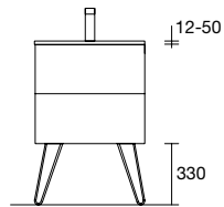
PÉS PARA LAVATÓRIOS INTEGRAIS ALTURA 330 mm
