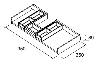
GAVETA COM ABERTURA PARA SIFÃO, DIREITA
