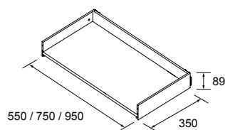
GAVETA METÁLICA SEM ABERTURA PARA SIFÃO
