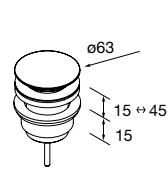
VÁLVULA ABERTA FLOW
