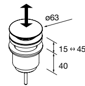
VÁLVULA CLICKER FLOW
