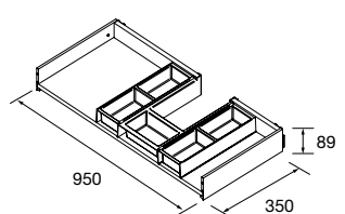
GAVETA COM ABERTURA PARA SIFÃO, ESQUERDA
