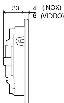
Versão mecânica
